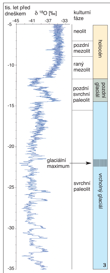
3 Chronostratigrafická tabulka s vyznačením všech zmiňovaných období; δ 18 O je podíl množství izotopů 18 O a 16 O ve vzorku z Grónského ledovce (GRIP) ve vztahu k množství izotopů 18 O a 16 O obsažených ve standardu – vyšší hodnota souvisí s vyšší teplotou. Orig. P. Kuneš
